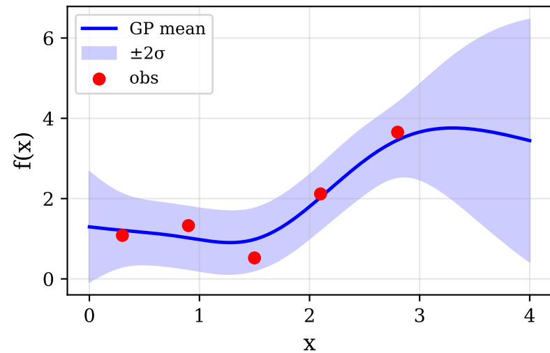
(a) GP posterior
